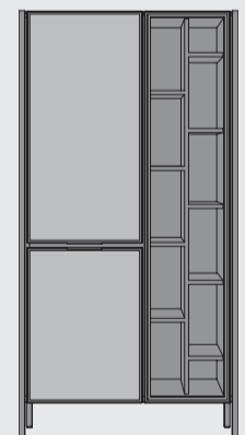
Schrank B95 x T44 x H190 cm 2 Türen + 11 Nischen (+LED) art: 40648
