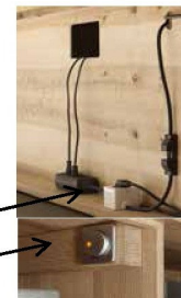
ALL ON/ ALL OFF Schalter
